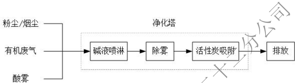
图 3 废气处理工艺流程图
