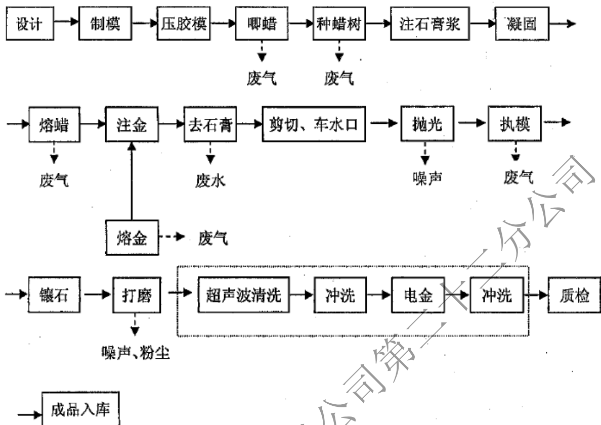
图1 原有项目的生产工艺流程图示意图（引自原有项目环评文件）
