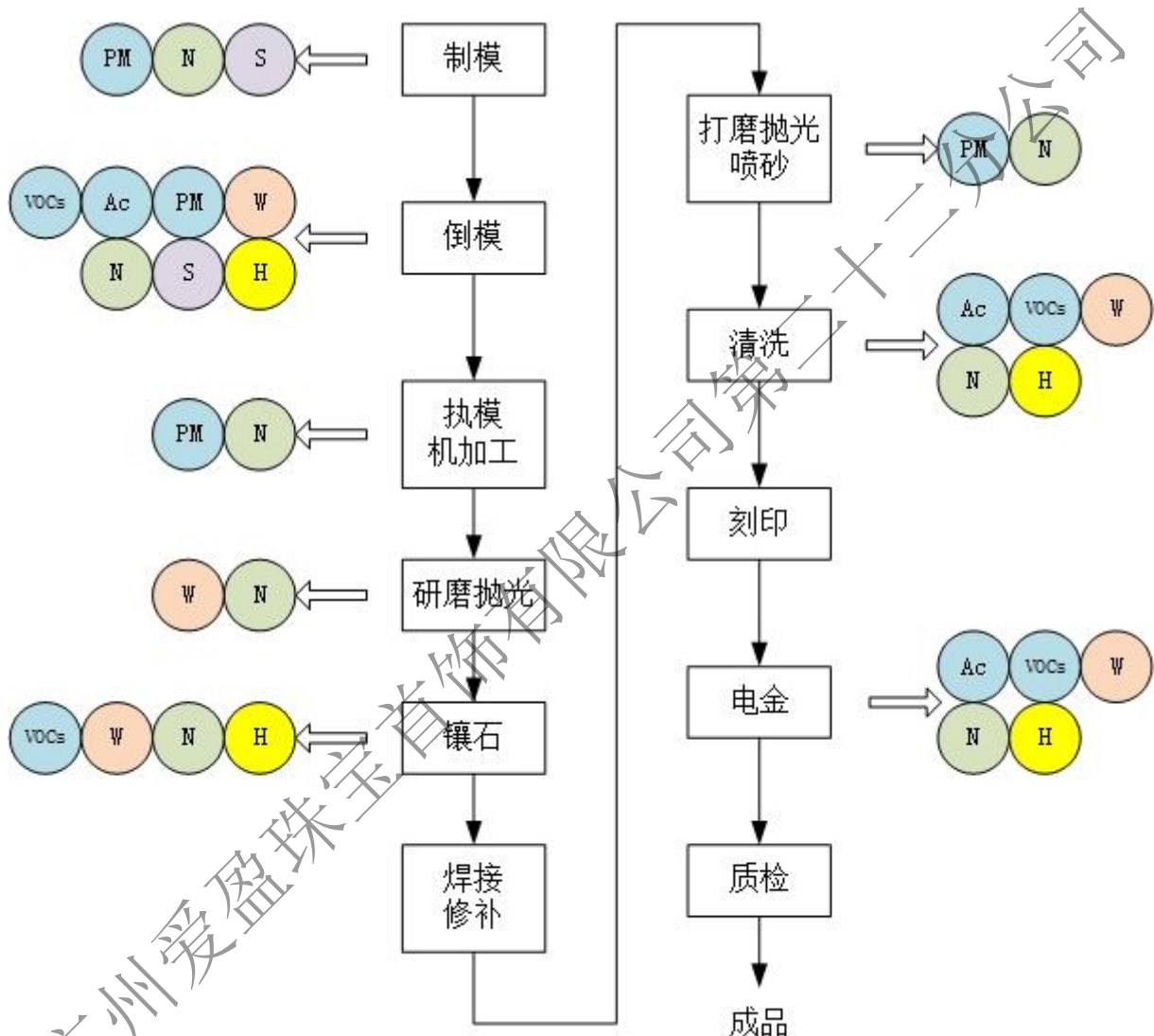
图 2 工艺流程和产污环节示意图
