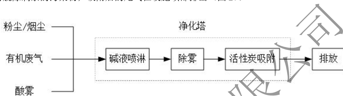
图 2 废气处理工艺流程图
