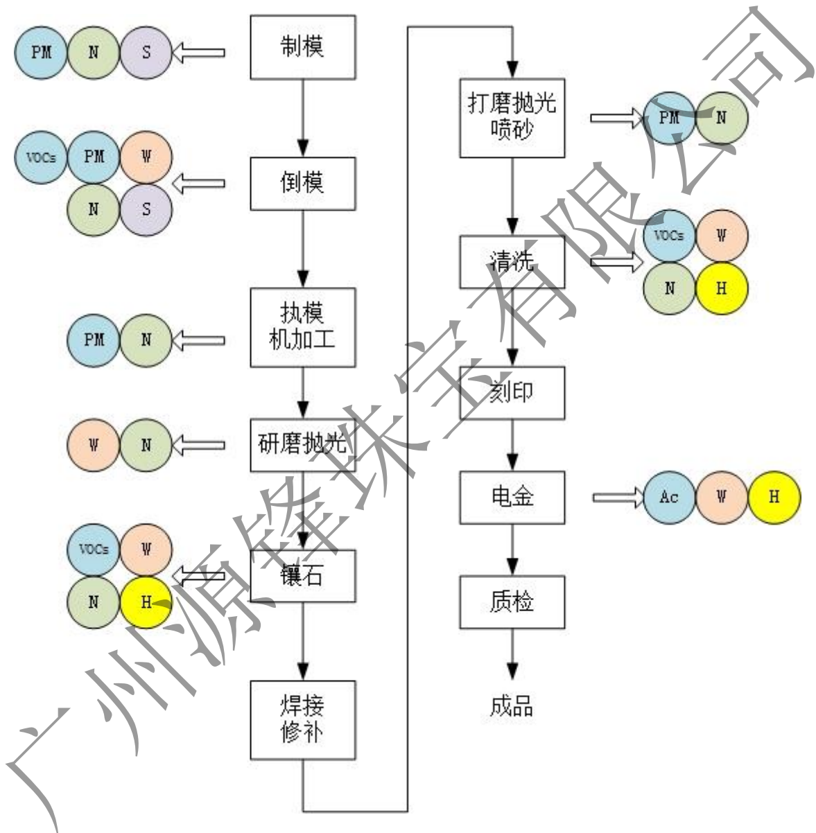
图 1 工艺流程和产污环节示意图
