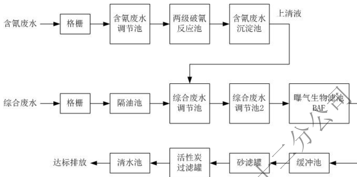
图3 产业园废水处理工艺流程图
